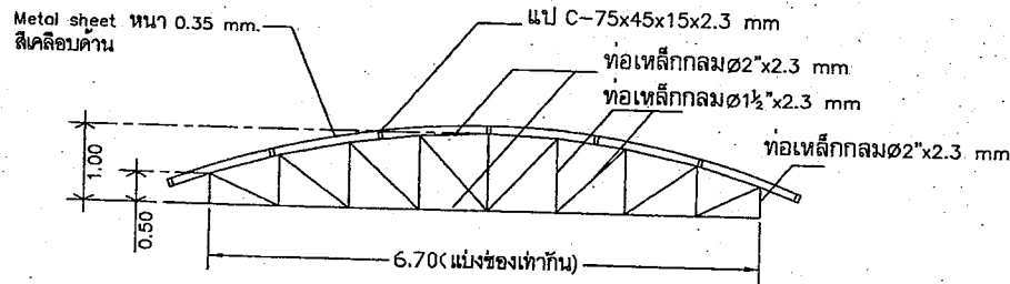
แบบขยายหลังคาจุดที่2 TRUSS (T1)
