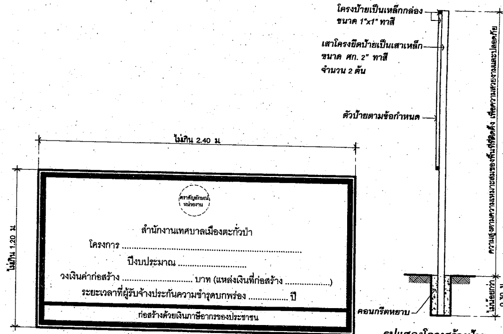
รูปแสดงโครงสร้างป้าย
