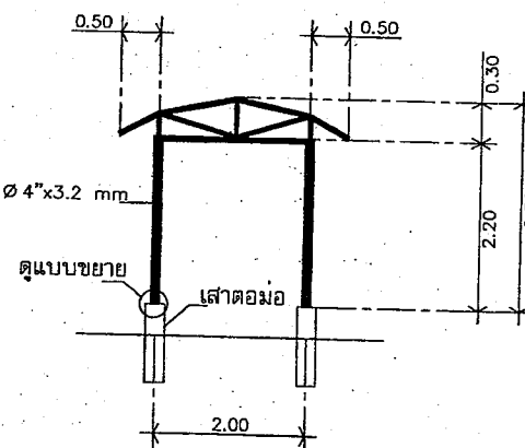
รูปตัดหลังคา จุดที่ (3.1) (3.2)
