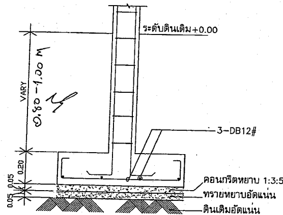
F2 SCALE 1 : 20
