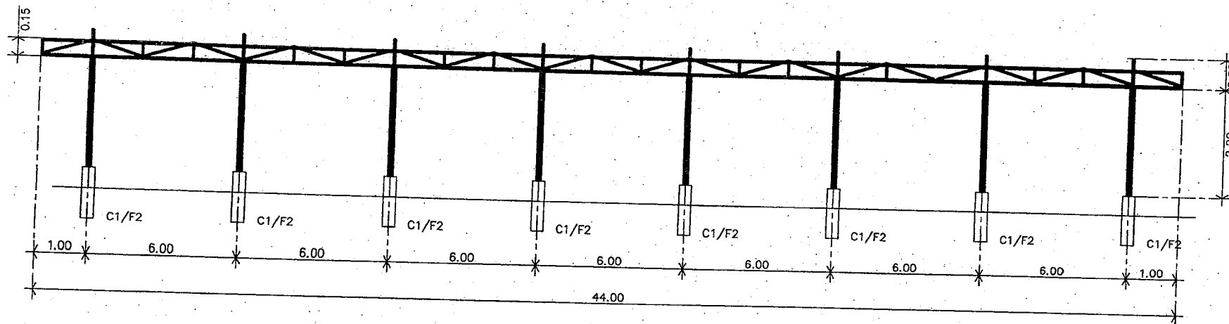
รูปตัดหลังคา จุดที่ (3.1)
