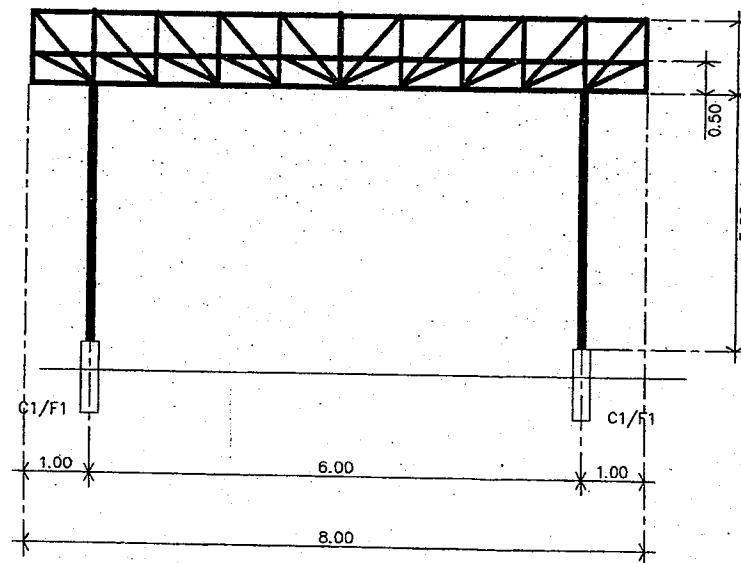
รูปตัดหลังคา จุดที่ ④
