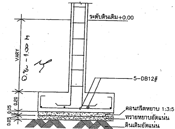
F1 SCALE 1 : 20
