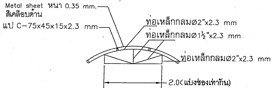
แบบขยายหลังคาจุดที่ 3.1 TRUSS (T3)
