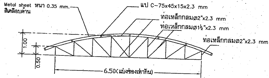
แบบขยายหลังคาจุดที่1 TRUSS (T1)
