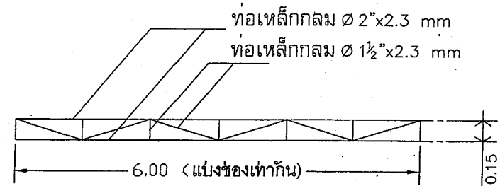
แบบขยายหลังคาจุดที่ 3.1 TRUSS (T4)
