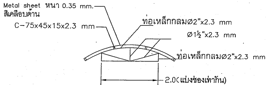
แบบขยายหลังคาจุดที่ 3.2 TRUSS (T3)
