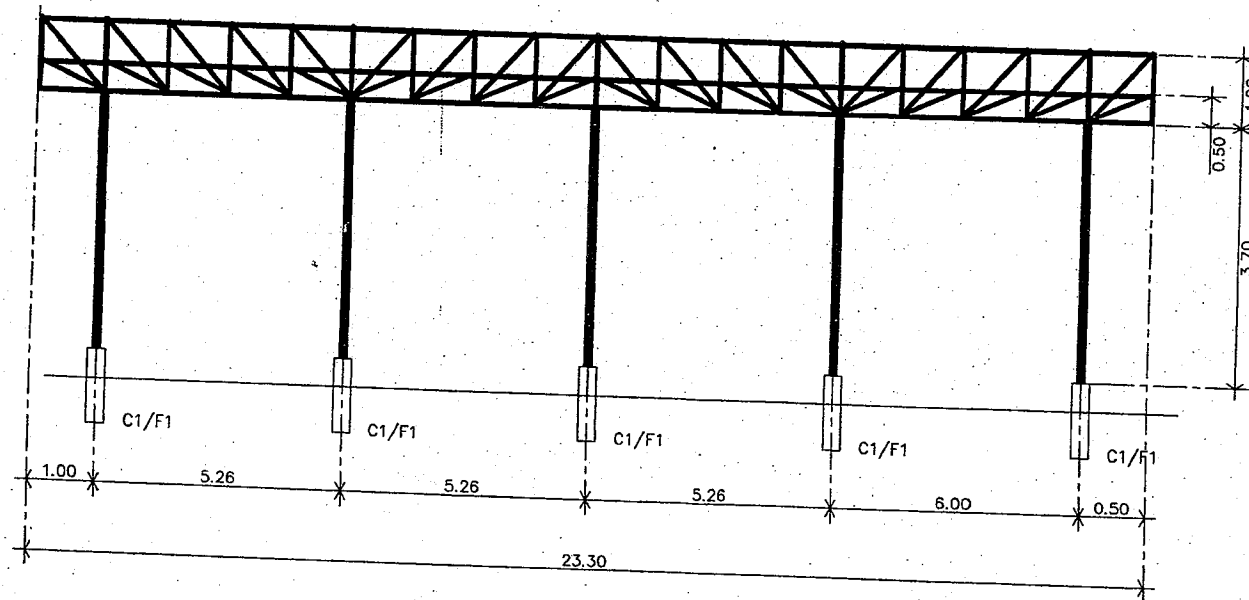
รูปตัดหลังคา จุดที่ ②
