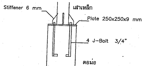
แบบขยายฐานเสา
