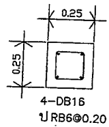
แบบขยายเสาตอม่อ C1
