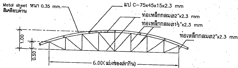
แบบขยายหลังคาจุดที่4 TRUSS (T1)
