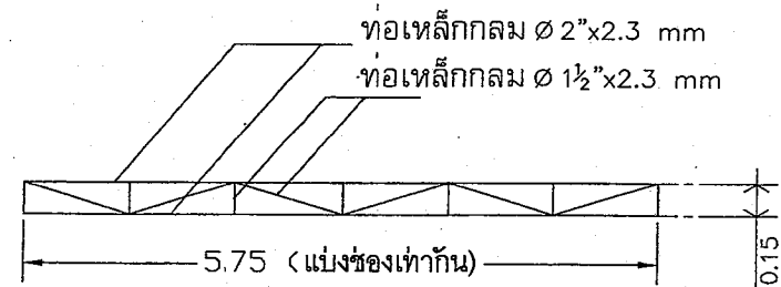
แบบขยายหลังคาจุดที่ 3.2 TRUSS (T4)
