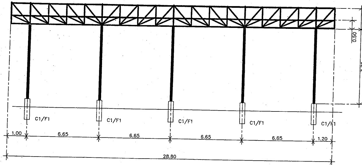
รูปตัดหลังคา จุดที่ ①
